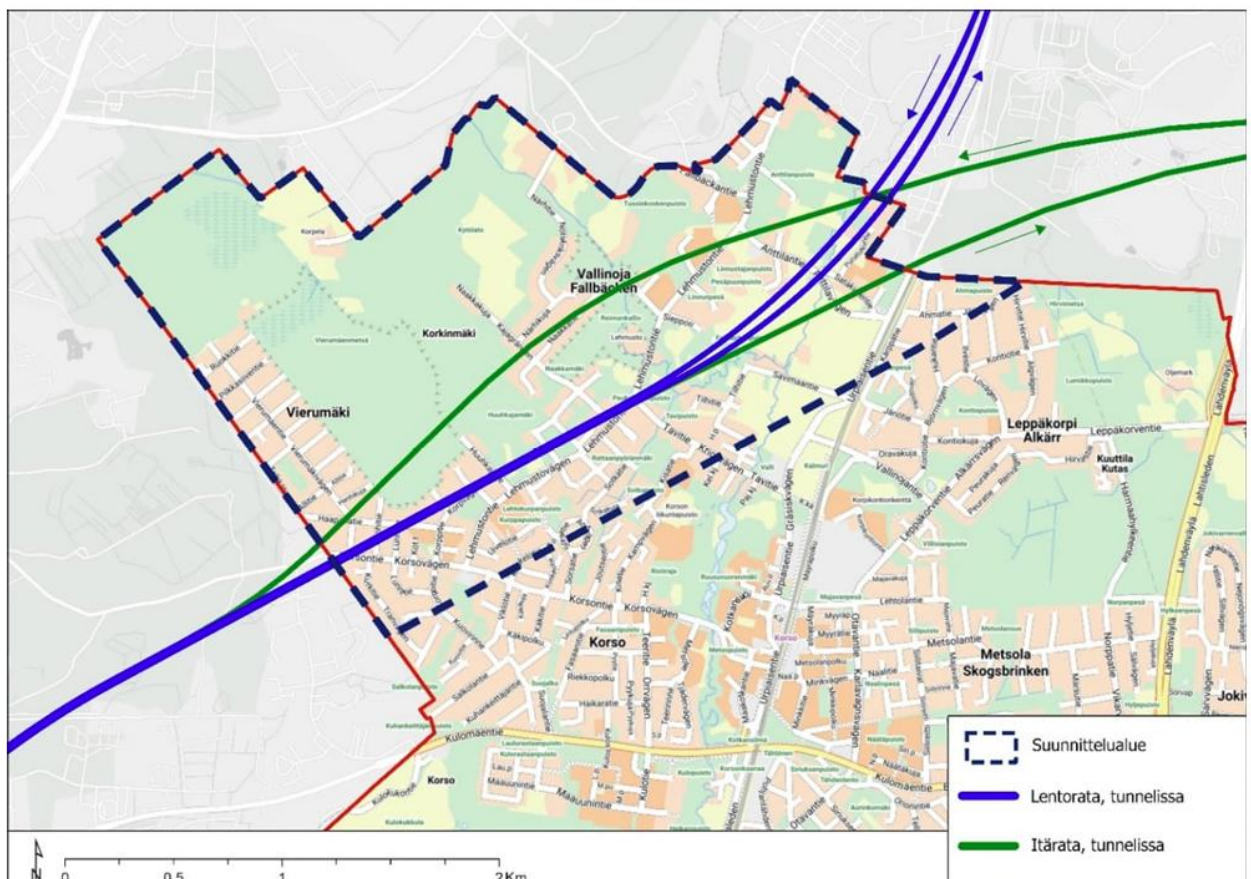
Kuva 1. Itäradan ja Lentoradan ratatunnelit suunnittelualueella.
